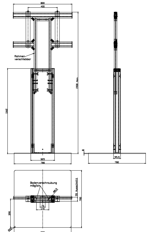
UniversAL BS-46 hier mit 65" LCD
